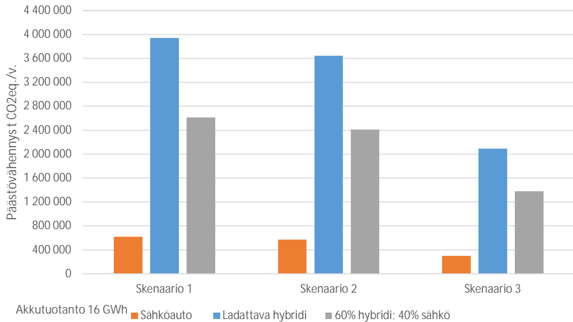
Kuva 3. Päästövähennys (t CO2eq./v.) suhteessa vastaavaan määrään polttomoottoriautoja kun akkutuotantokapasiteetti 16 GWh/a.
