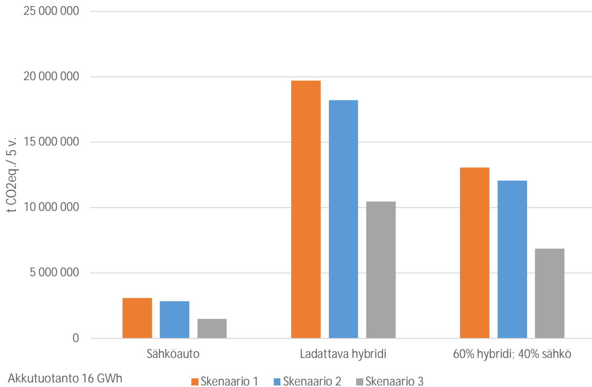
Kuva 4. Päästövähennys (t CO 2 eq.) laskettuna viidelle vuodelle kun akkutuotantokapasiteetti 16 GWh/a.
